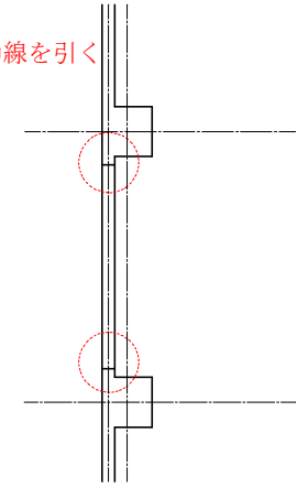
⑤建具の作図-2（壁線の追加）
